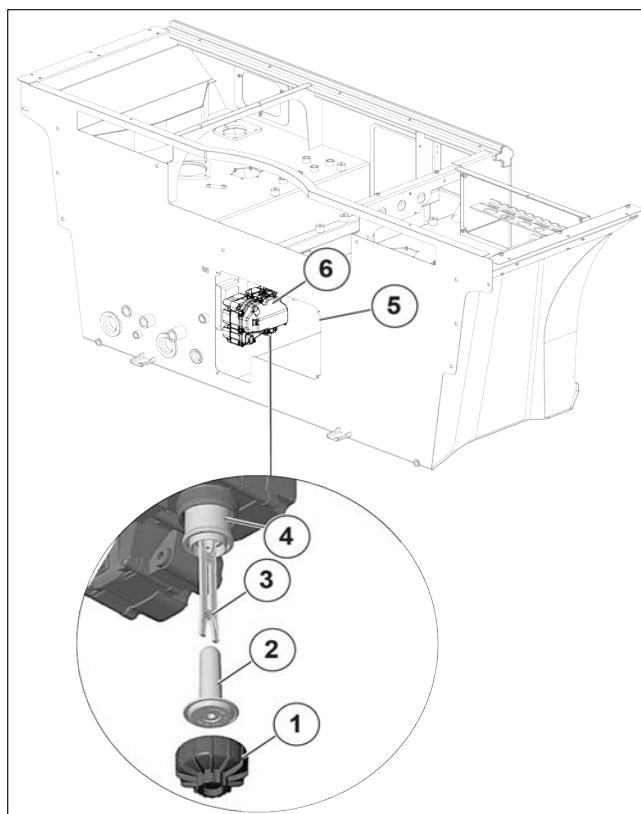
Figure 204: Remplacement du filtre de la pompe de gavage « DEF »
