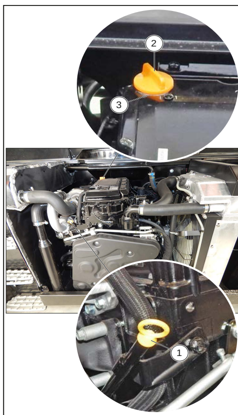
Figure 144: Niveau d'huile moteur
