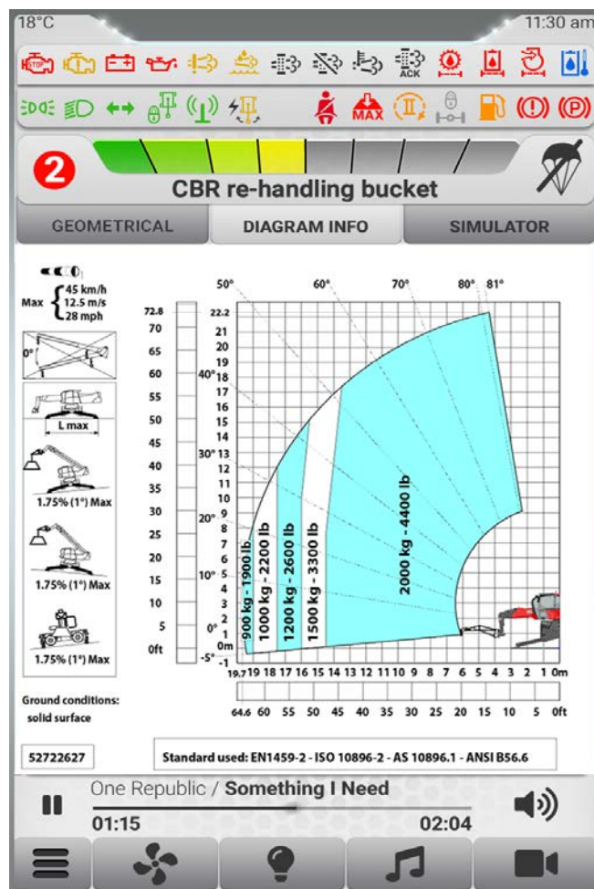
Figure 87: Onglet « INFO DIAGRAMME »
