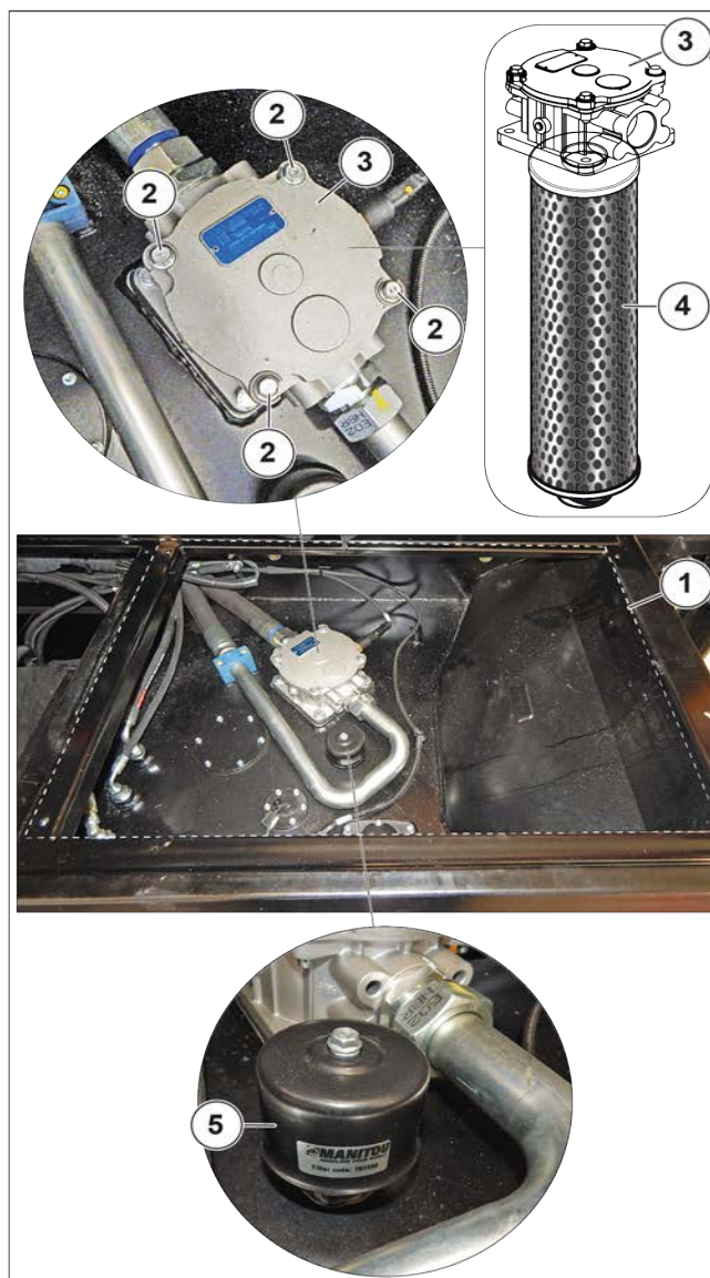
Figure 176: Remplacement du reniflard d'huile hydraulique
