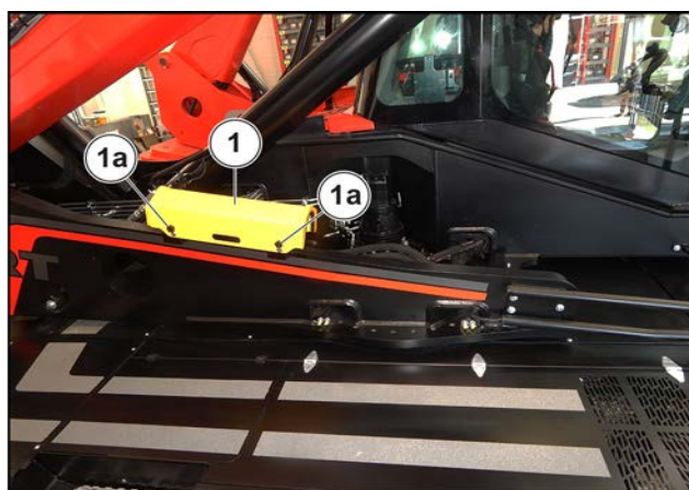
Figure 67: Cale de sécurité de la flèche
