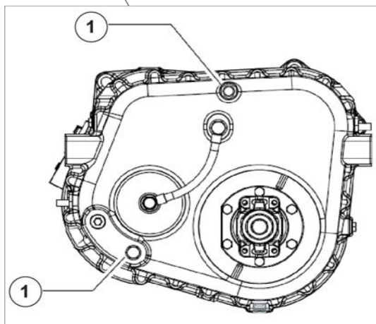
Figure 164: VÉRIFICATION DU NIVEAU D'HUILE DE LA BOÎTE DE VITESSES
