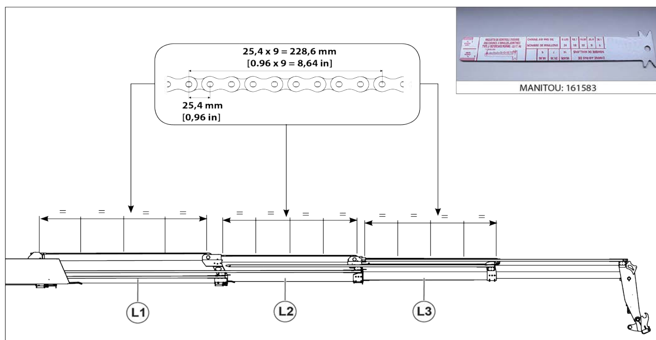
Figure 198: Allongement des chaînes
