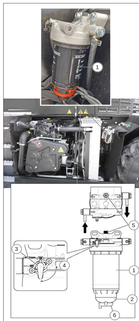
Figure 150: Vérification du préfiltre à carburant
