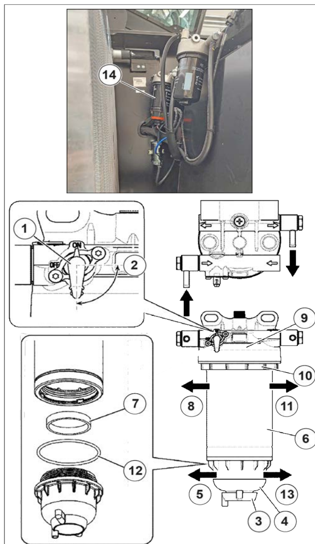
Figure 188: Remplacement du préfiltre à carburant
