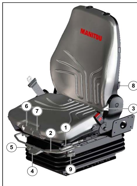
Figure 70: Siège pneumatique pour le conducteur (en option)
