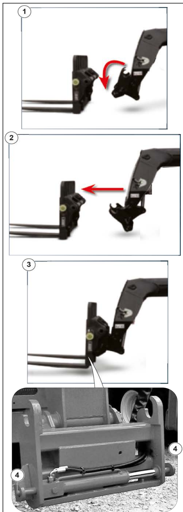
Figure 124: Repose de l'accessoire avec bloc hydraulique (en option)
