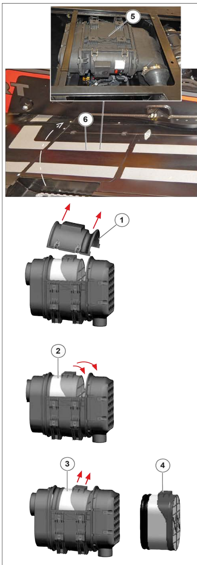
Figure 186: Remplacement de la cartouche de filtre à air sec
